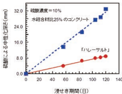
濃度10%の硫酸による浸せき試験結果
