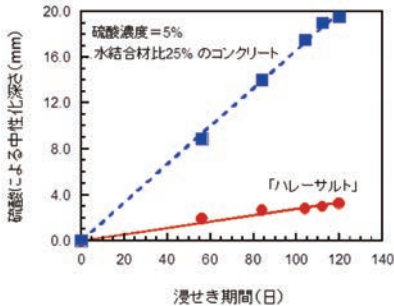
濃度5%の硫酸による浸せき試験結果
