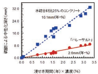
浸せき期間と濃度の積と硫酸による中性化深さの関係
